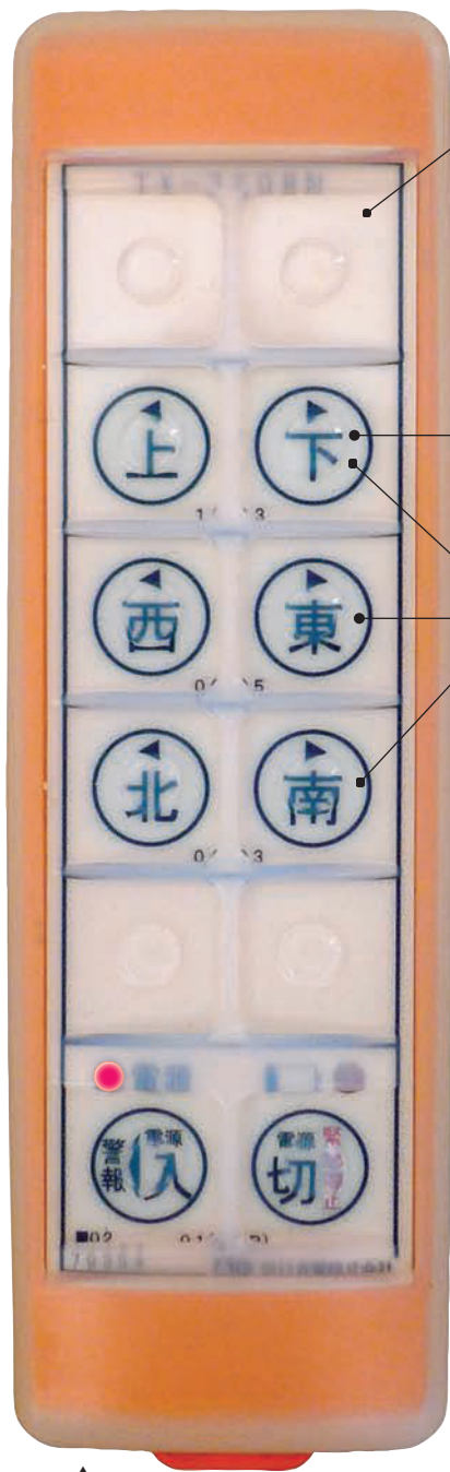
チップケーブルレス送信機 TX-3208N (原寸大) 175×52×32mm 200g
